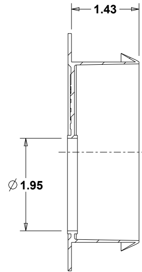
SECTION A-A
